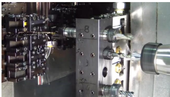
Pracovní prostor dlouhotočného automatu Manurhin z TAJMAC-ZPS a ukázka virtuálního simulačního modelu stroje.
