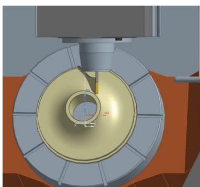
Pracovní prostor dlouhotočného automatu Manurhin z TAJMAC-ZPS a ukázka virtuálního simulačního modelu stroje.
