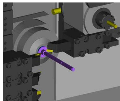
Pracovní prostor dlouhotočného automatu Manurhin z TAJMAC-ZPS a ukázka virtuálního simulačního modelu stroje.
