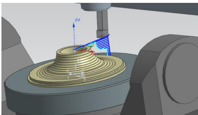
Základní technologické možnosti stroje KOVOSVIT MAS MCU700VT-5X, které vyvinutý postprocesor umožňuje plně využít – frézování, soustružení karuselováním, soustružení s naklopenou osou A, soustružení s plynulým naklápěním osy A.
